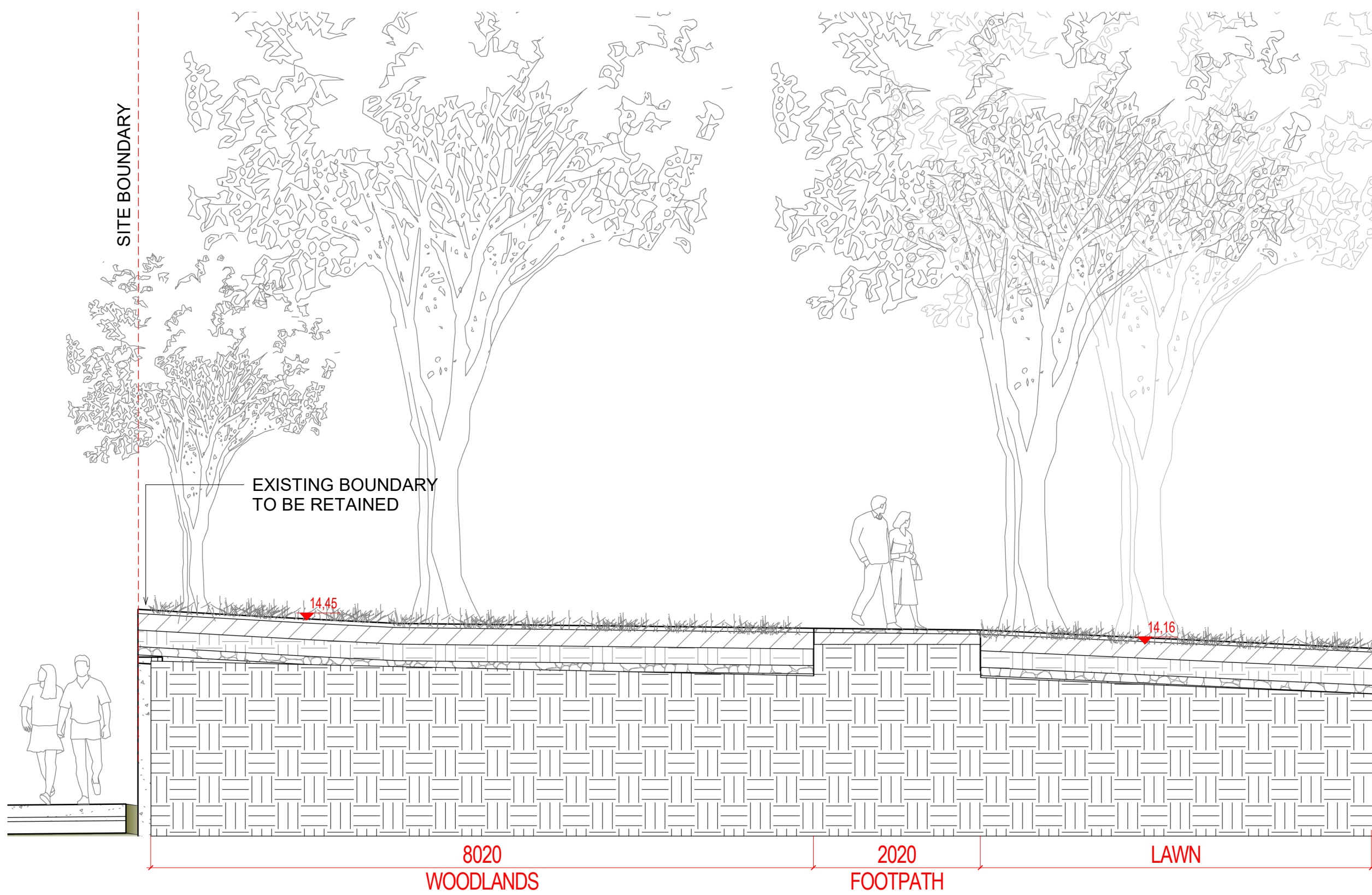
2 SECTION 47 1:50 @A1
