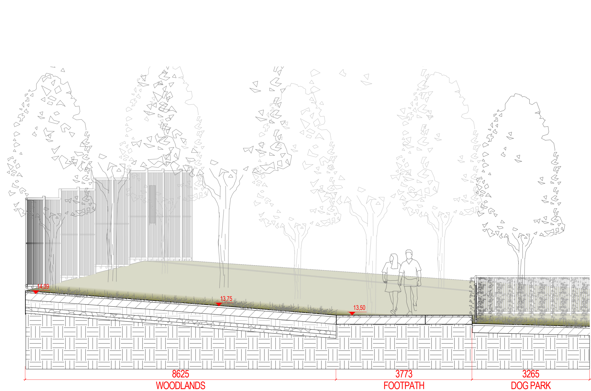
1 SECTION 46 1:50 @A1
