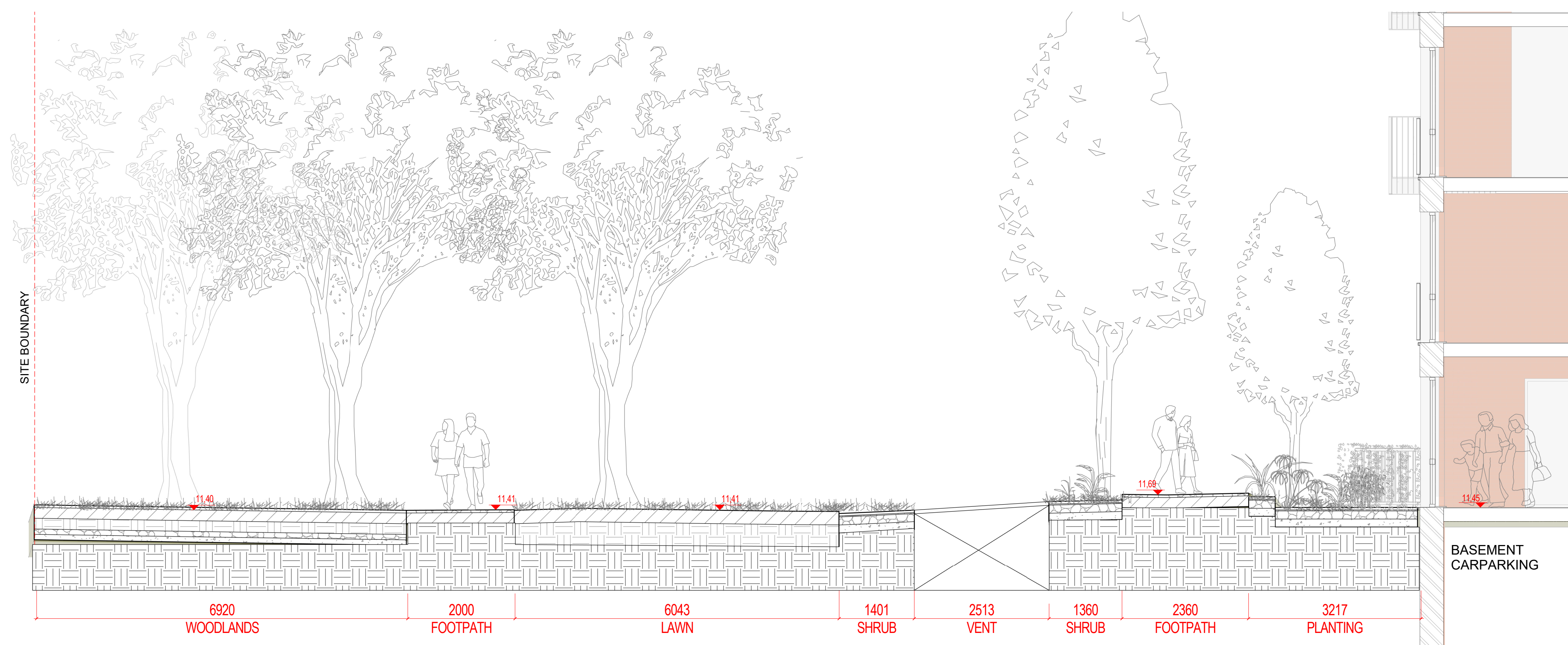
3 SECTION 48 1:50 @A1
